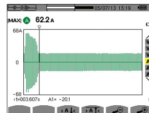
Inrush-Funktion
