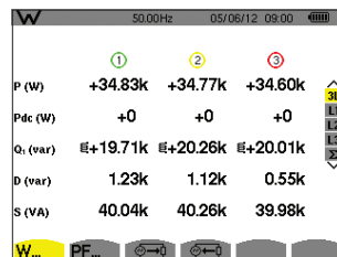
Leistungsmessung
