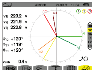
Phasendiagramm
