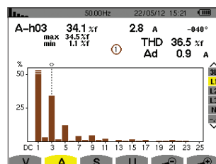
Oberschwingungsanalyse
