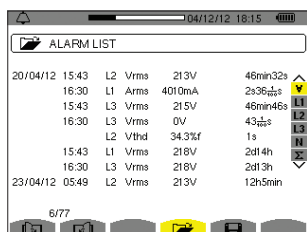
Alarm-Funktion
