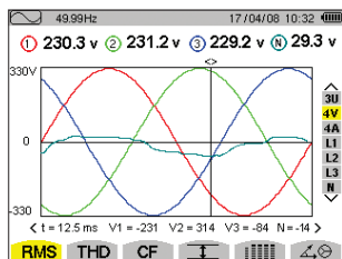
Scope-Funktion
