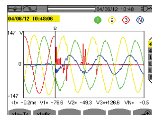
Transientenerfassung
